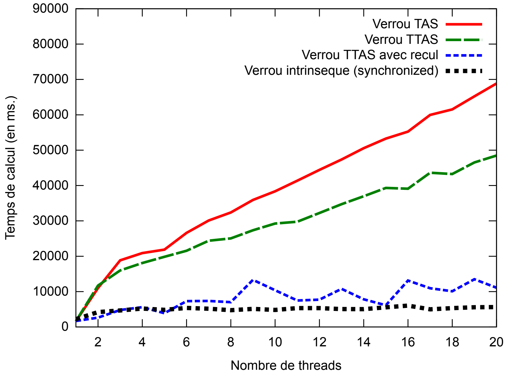
Performances des verrous pour les compteurs anarchiques
